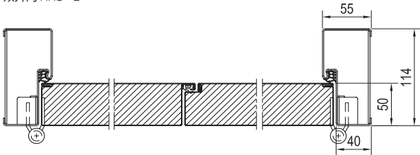
双开门 HHS - 2
